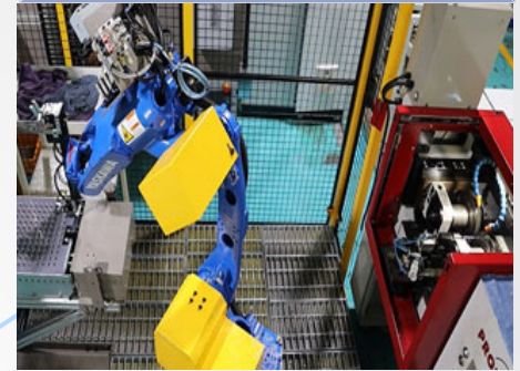
3 Block (전조)
