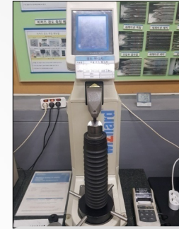
로크웰 경도기
